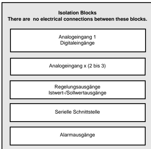
Abbildung 8.5 — Galvanische Trennung.
