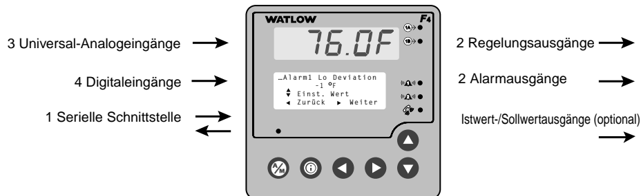
Abbildung 1.1 — Ein- und Ausgänge der Serie F4P (Standard-Regelung, 1 Eingang, F4P _ - _ _ AA - _ _ _ _; Erweiterte Regelung, 3 Eingänge, F4P _ - _ _ AB - _ _ _ _).
