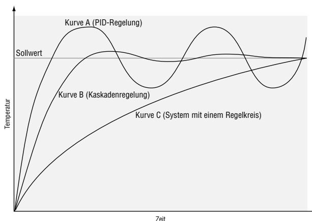
Abbildung 7.15a — Regelungsverzögerungen.
