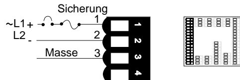
Abbildung 8.5 — Netzanschluß.
