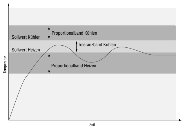
Abbildung 7.7c — Toleranzband Kühlprozeß.
