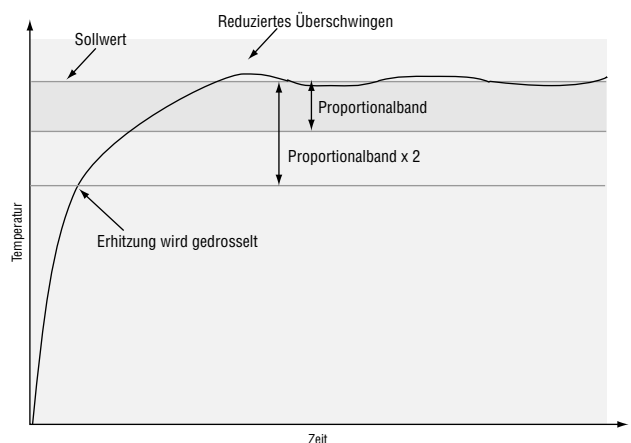
Abbildung 7.7b — PID-Regelung.
