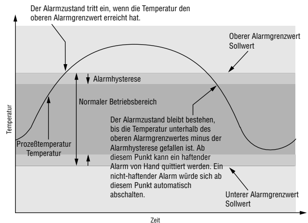
Abbildung 7.11a — Haftender Alarm.
