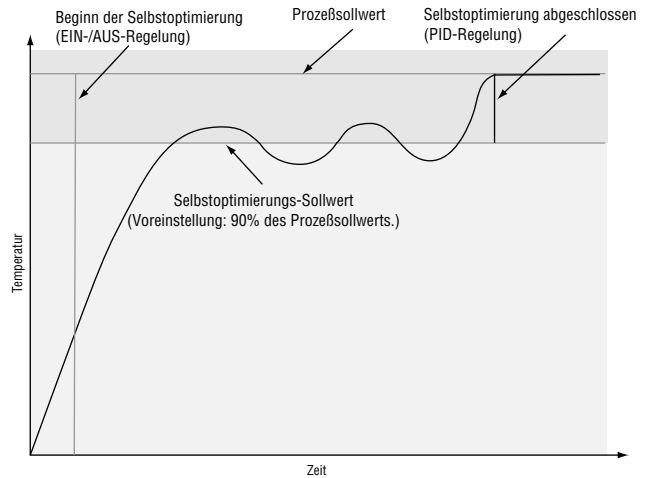
Abbildung 7.9 — Selbstoptimierung
