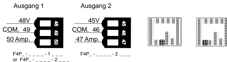
Abbildung 8.11c — Alarmausgang x (1 und 2)
