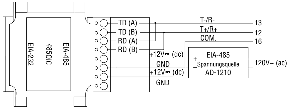
Abbildung 8.13 — Umwandlung EIA/TIA 232 in EIA/TIA 485
