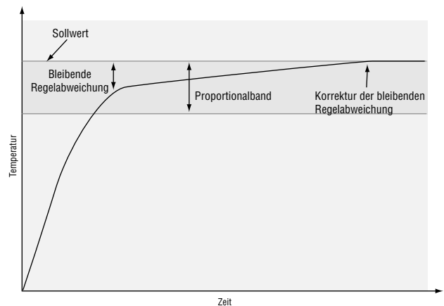
Abbildung 7.7a — Proportional- plus Integralregelung.
