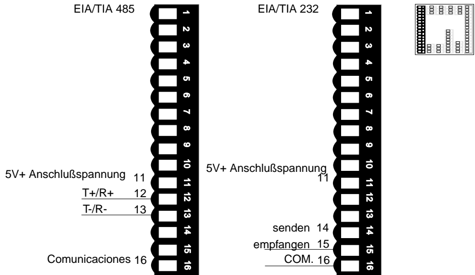
Abbildung 8.12a — Serielle Schnittstelle EIA/TIA 485 und EIA/TIA 232
