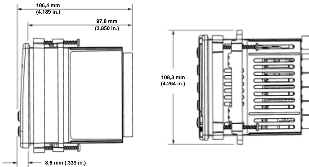
Abbildung 8.2a — Abmessungen der Seitenansicht und der Geräteoberseite.
