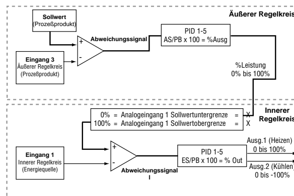
Abbildung 7.15b — Kaskadenregelung.
