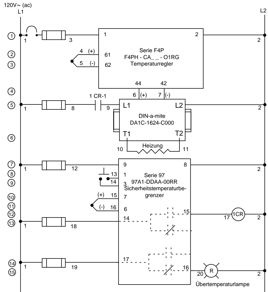
Abbildung 8.14 — Verdrahtungsbeispiel eines Systems.
