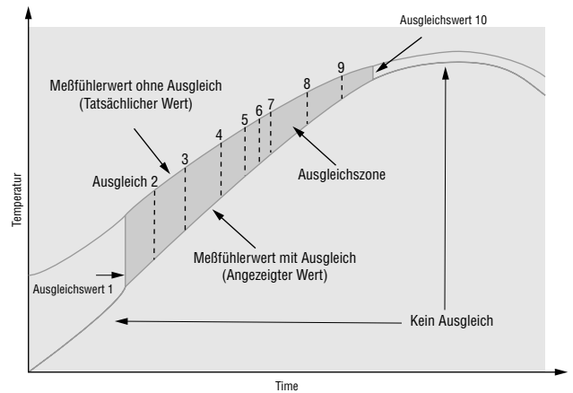
Abbildung 7.2 — Verwendung mehrerer Ausgleichspunkte.
