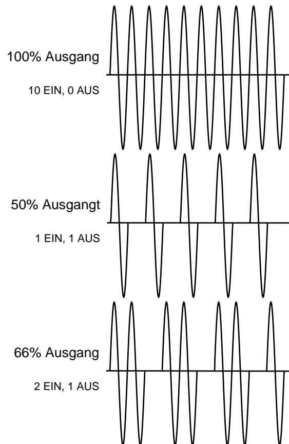
Abbildung 7.8b — Impulsgruppenregelung
