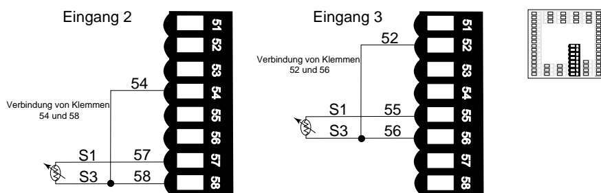
Abbildung 8.7c — Pt-100 (in 3-Leiterschaltung)
